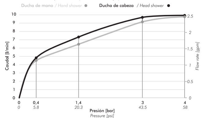
Gráfico de caudales de operación / Operation flow rate graphic
